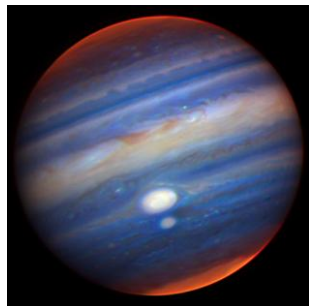
Planétologie
