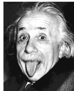
Relativité
