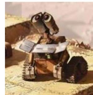
Systèmes embarqués
