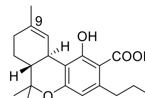
THCVA
