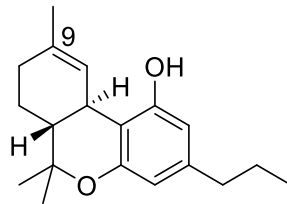
THCV
