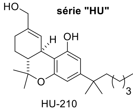
séries naphthoyl-indoles
