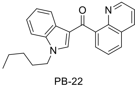
série quinoliny-indole
