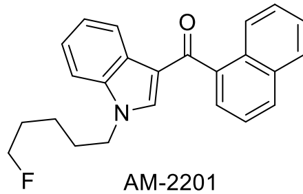
séries naphthoyl-indoles
