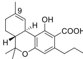
THCVA
