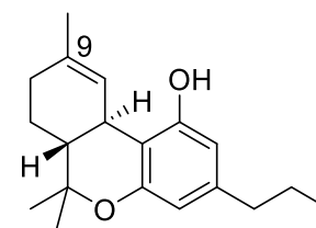
THCV
