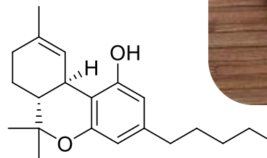
\Delta^9 -THC
