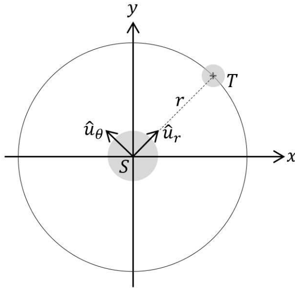
FIGURE 6.2 – Rotation d'une planète autour d'une étoile.
