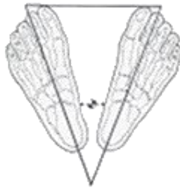
Base et triangle de sustentation, projection de la ligne de gravité du corps.
