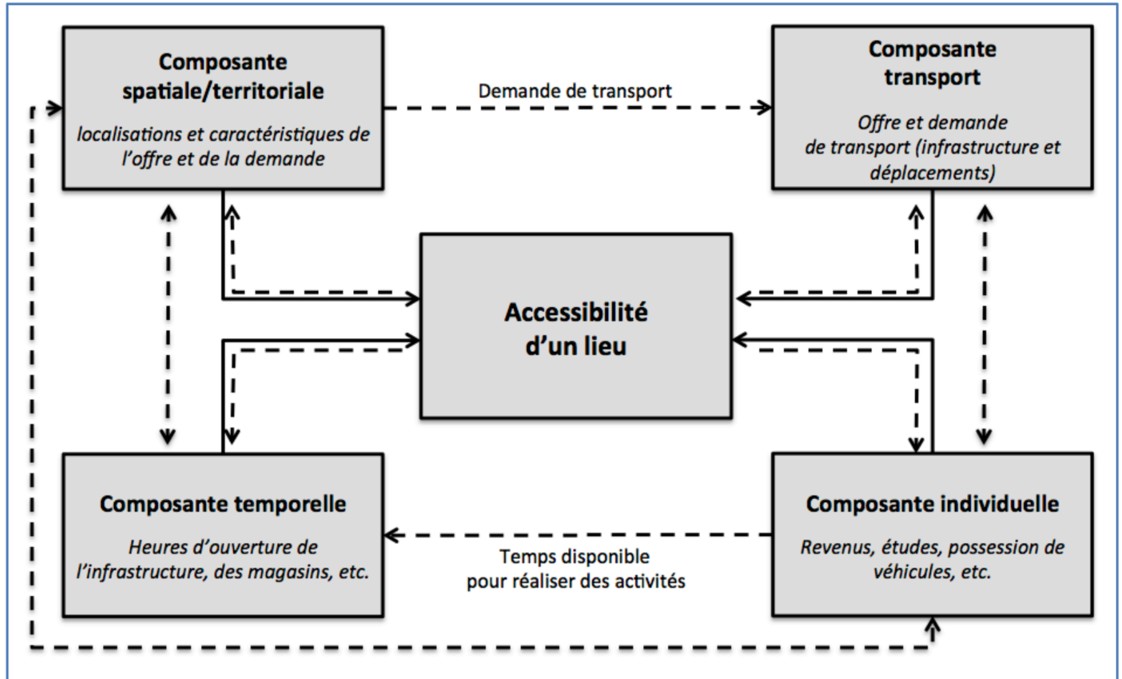
Figure 7 : Les relations entre les différentes composantes de l'accessibilité, d'après Geurs et Ritsema van Eck (2001 : 44)
